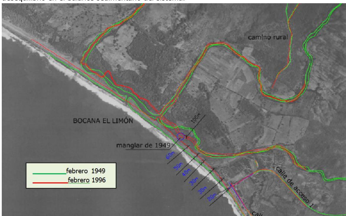
Figura 1. Superposición de bordes de playa y ríos para 1949 y 1996 sobre fotografía aérea de 1949.
