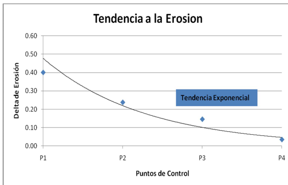
Gráfico 1. Línea de tendencia (Exponencial) de puntos P1, P2, P3 y P4 de control de corrimiento horizontal de línea de playa. Nótese que existe una marcada disminución en el avance erosivo cuando los puntos sea acercan a la zona de acantilados.
