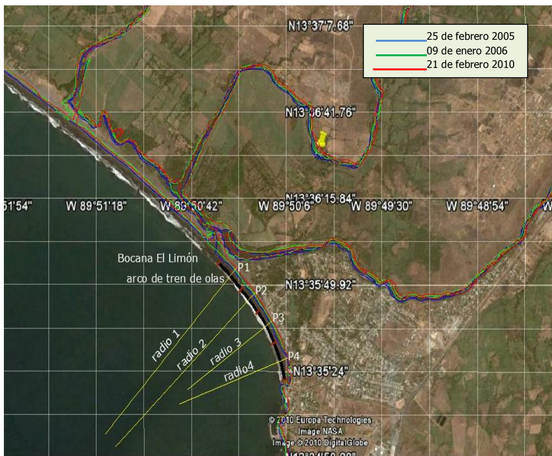
Figura 3. Arco de tren de olas y establecimiento de puntos P1, P2, P3 y P4 de control de corrimiento horizontal de línea de playa.
