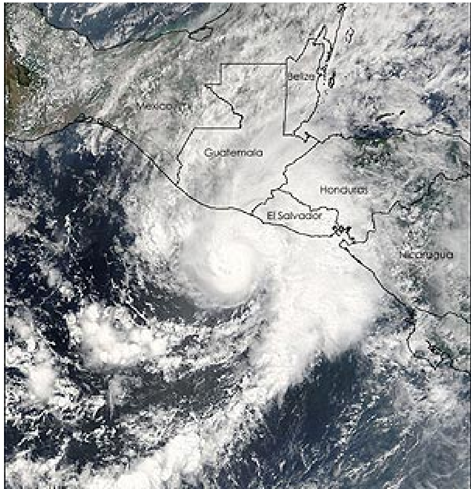
Fig. 9 Imagen del huracán Adrian tomada por la NASA (Foto: AP)
