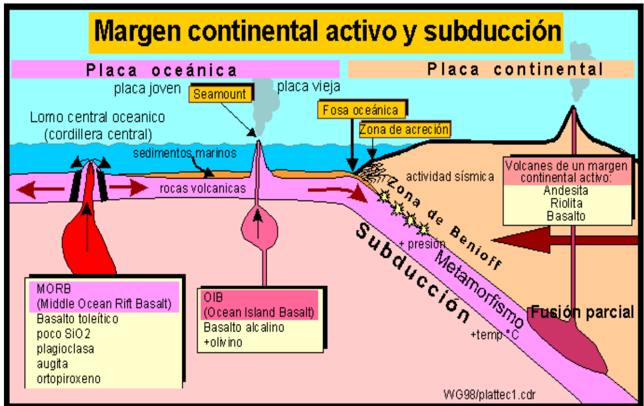
Fig. 2 Esquema del proceso de Subducción.
